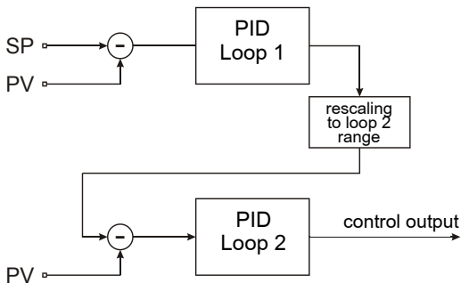
Fig. 24. Cascade control
