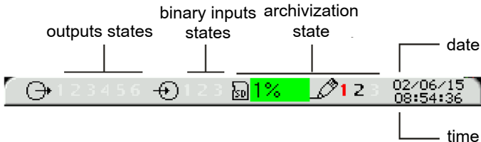
Fig. 4. Information bar
