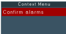
Fig. 16. Context menu
